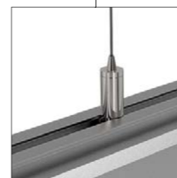
Подвес №10 для Т-образного паза (см. стр. 412)
